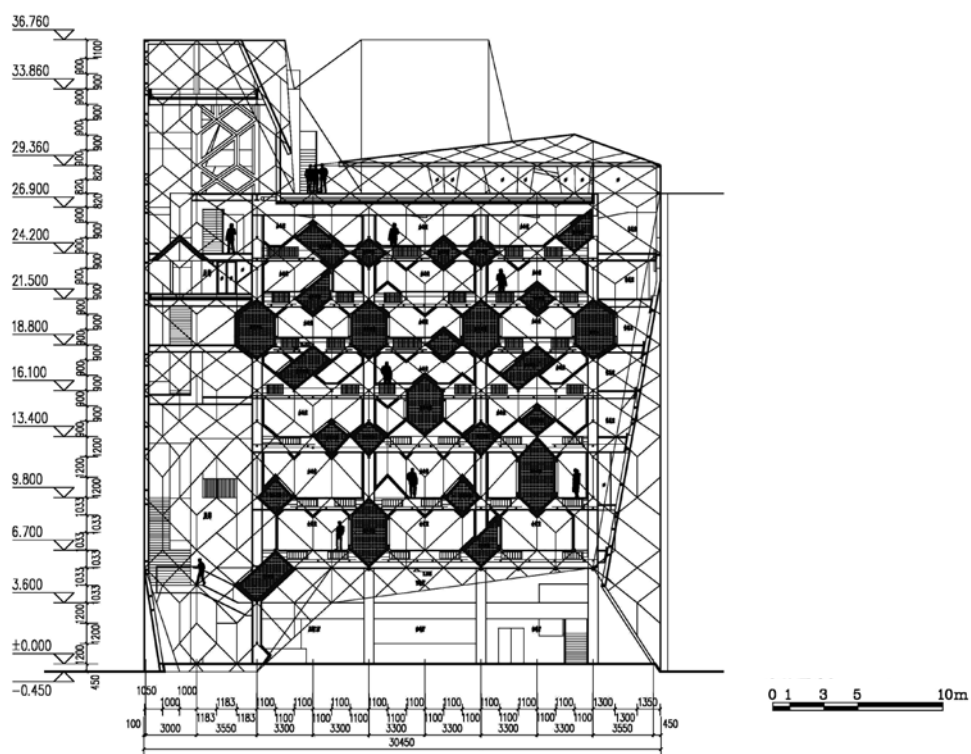
改造后剖面图
