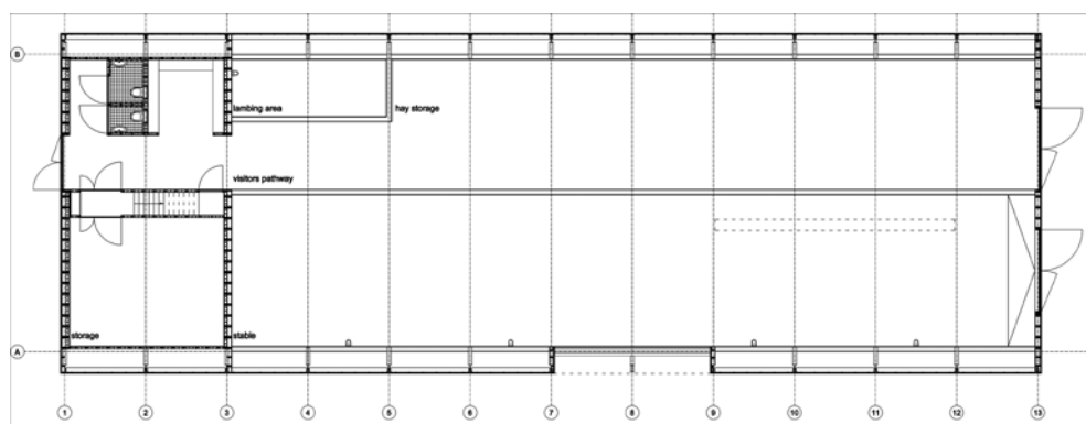
首层平面图面
