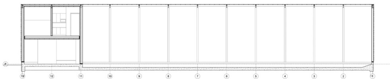
剖面
