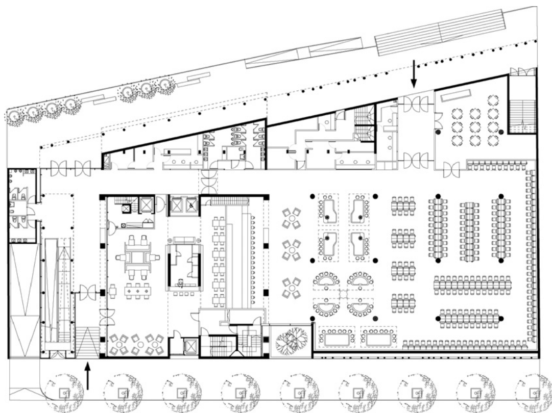
一层平面
