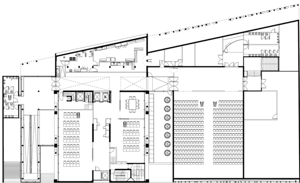
二层平面
