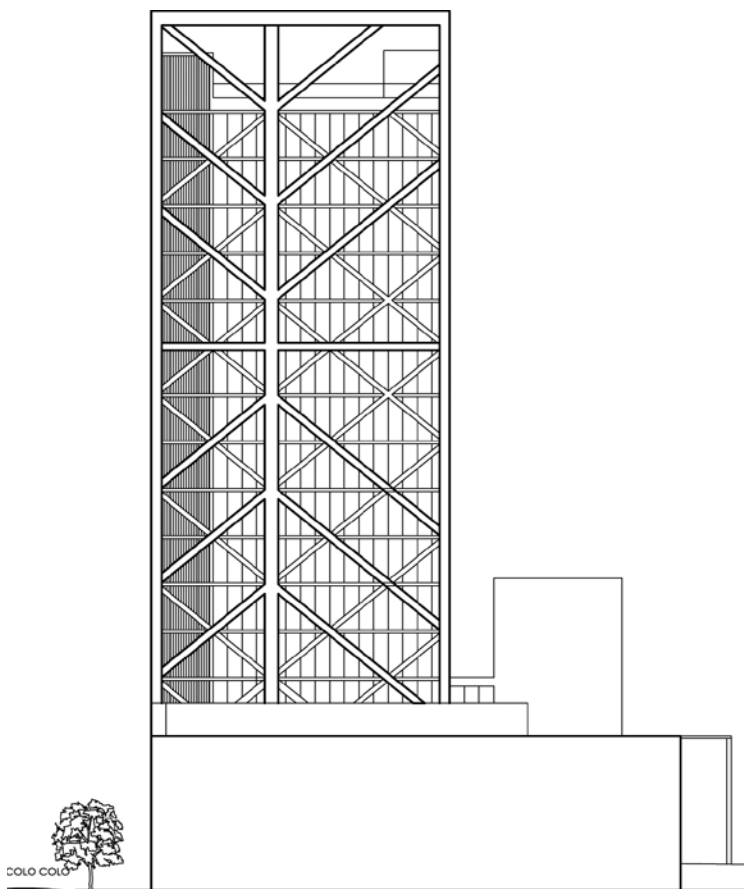
东立面
