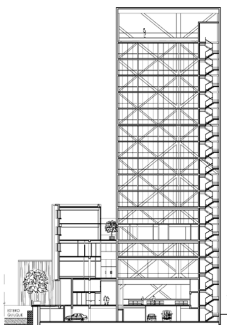
横剖面
