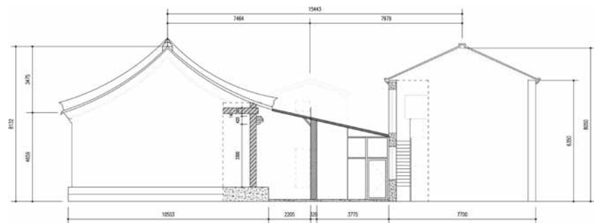
剖面图
