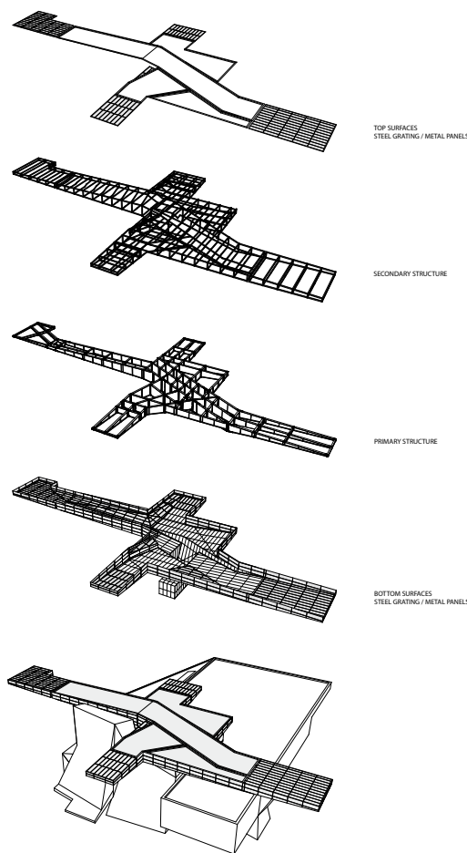
阿克伦博物馆屋顶层解构图
