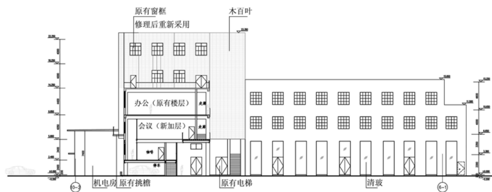
东立面图 (沿内院)
