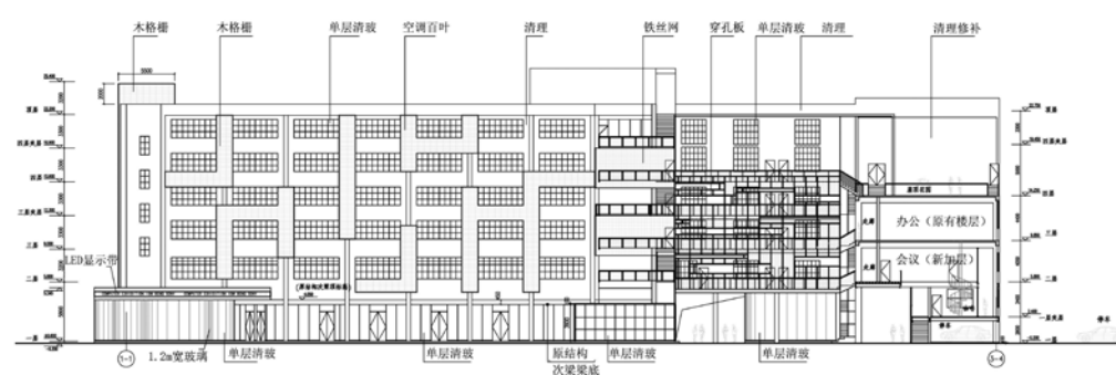
西立面图 (沿内院)
