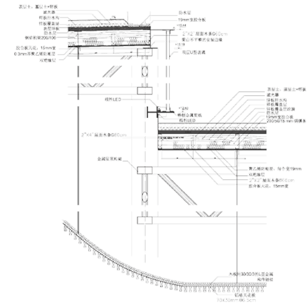
屋面及女儿墙剖面详图
