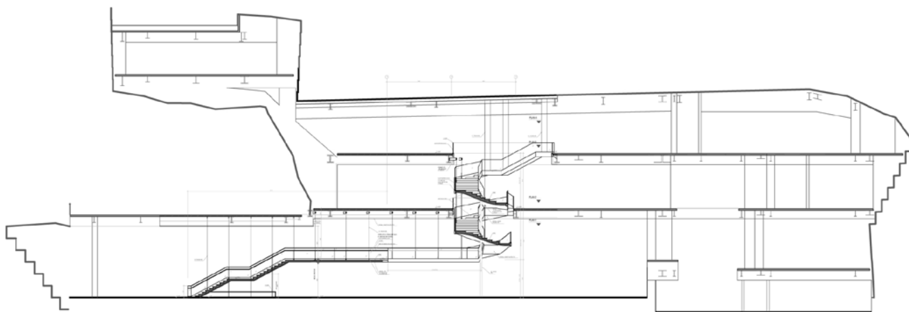
A-A剖面
