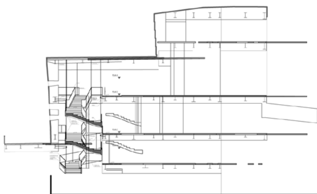
B-B剖面
