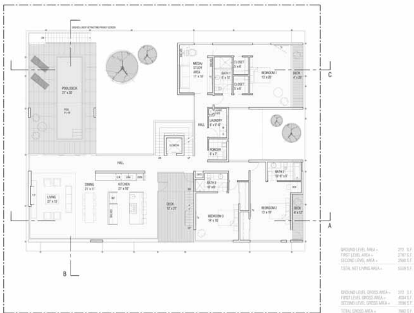
二层平面
