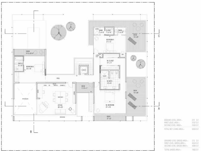
三层平面
