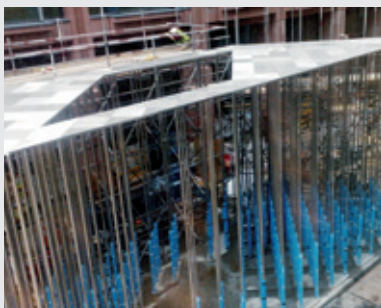
图8 正在建造中的装饰亭
