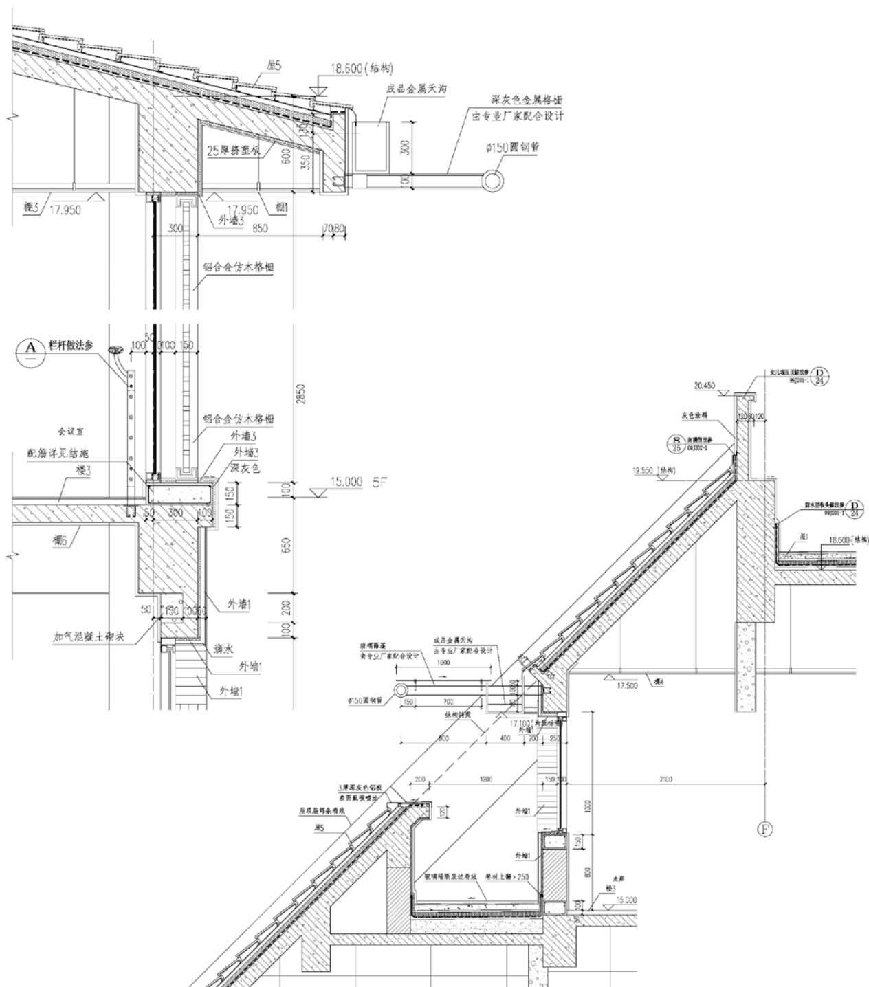
墙身大样
