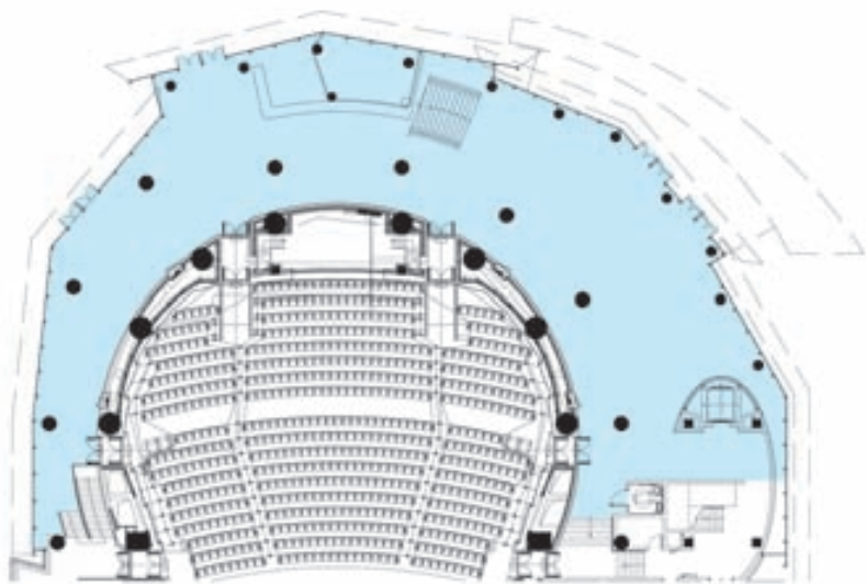
平面图
