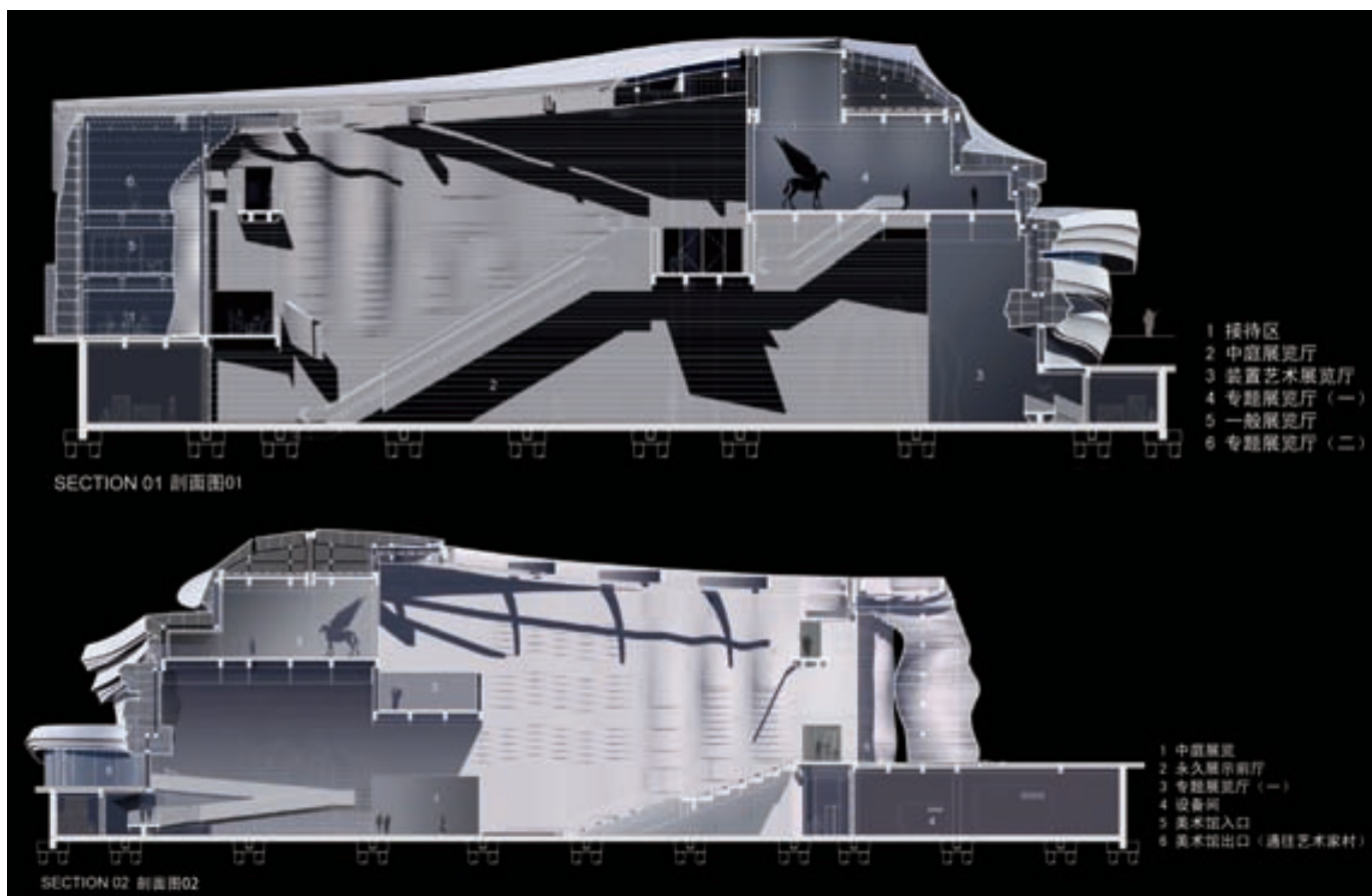
剖面图表达中庭部分
