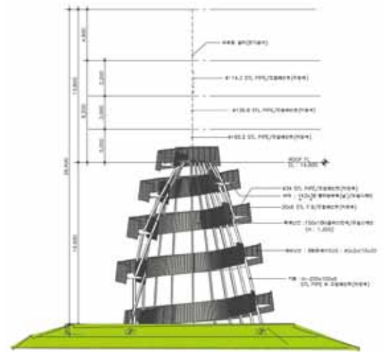
剖面图
