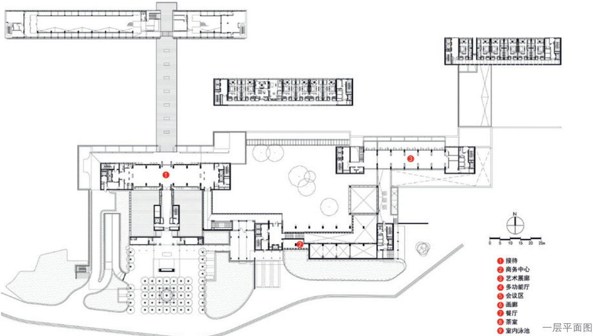
一层平面图
