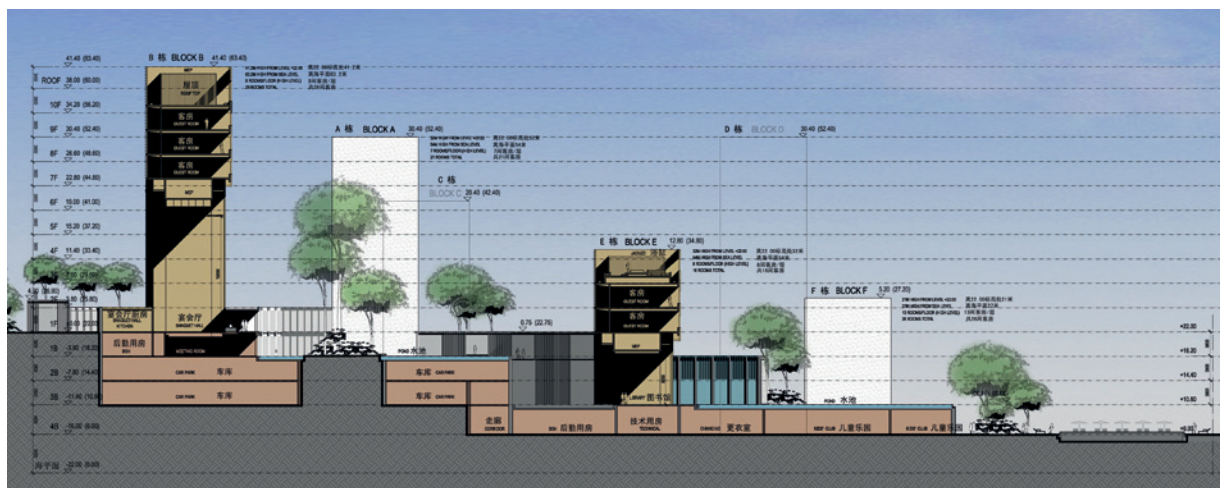
剖面图
